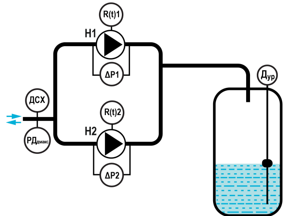
Рисунок 7.1 – Объект управления
