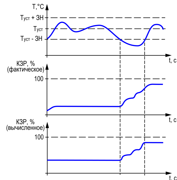
Рисунок 13.1 – Принцип работы КЗР
