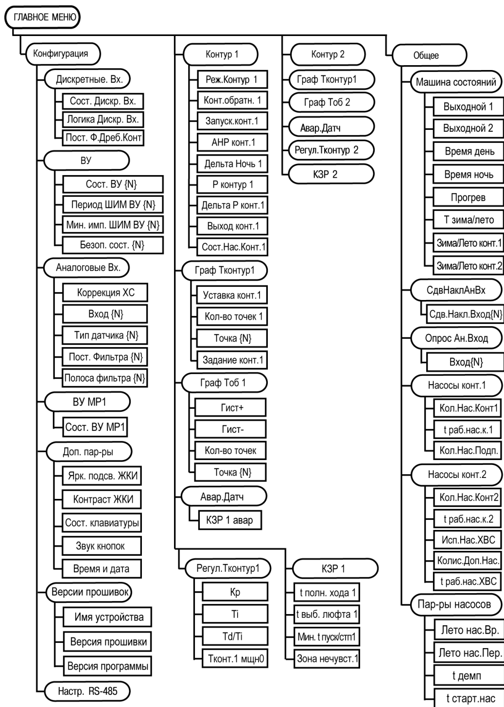
Рисунок 8.1 – Структура меню настройки
