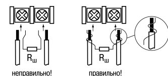
Рисунок 6.9 – Подключение датчиков с выходом в виде тока или напряжения
