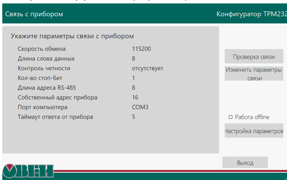
Рисунок 9.2 – Окно «Связь с прибором»
