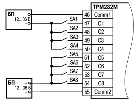
Рисунок 6.6 – Подключение датчиков к дискретным входам
