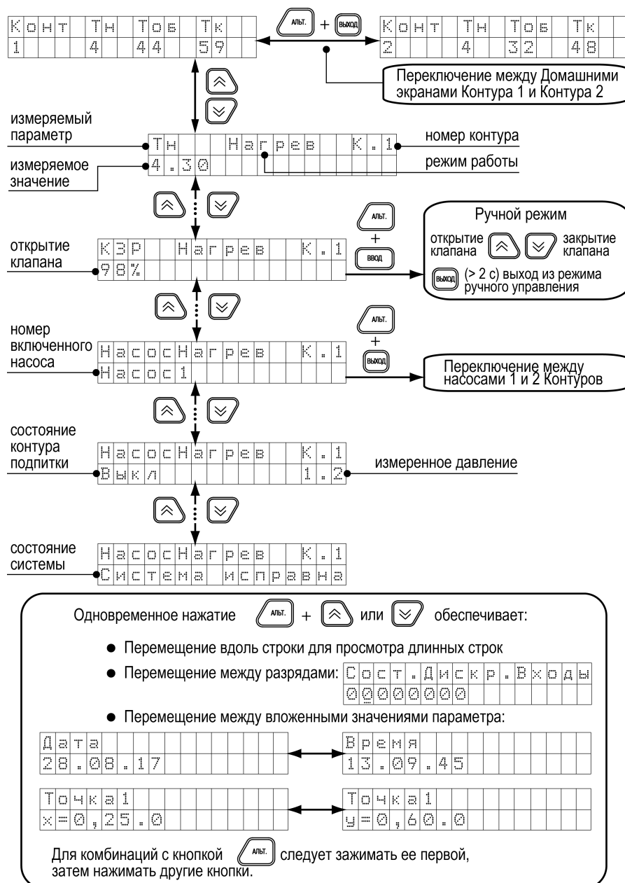
Рисунок 7.2 – Рабочие экраны 1
