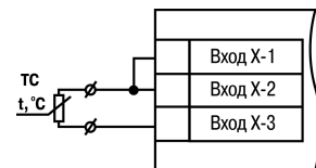
Рисунок 6.8 – Двухпроводная схема подключения ТС
