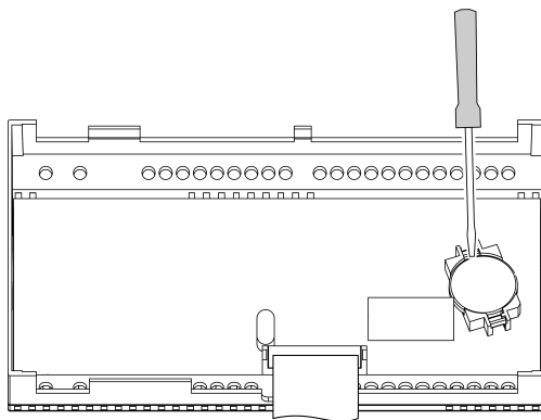
Рисунок 10.2 – Замена батарейки
