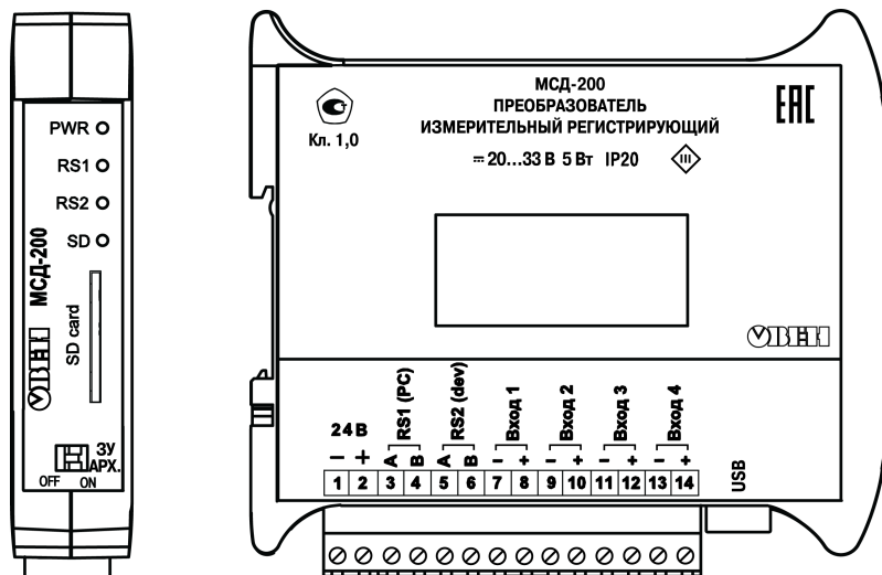
Рисунок 1.1 – Внешний вид прибора
