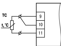
Рисунок 7 – Подключение ТС по трехпроводной схеме
